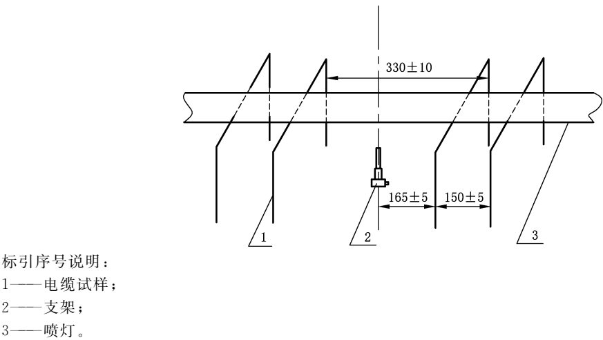
图 G.2 支架和喷灯位置
