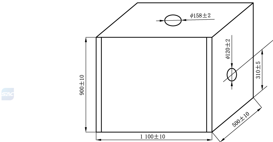
图 G.1 燃烧箱
