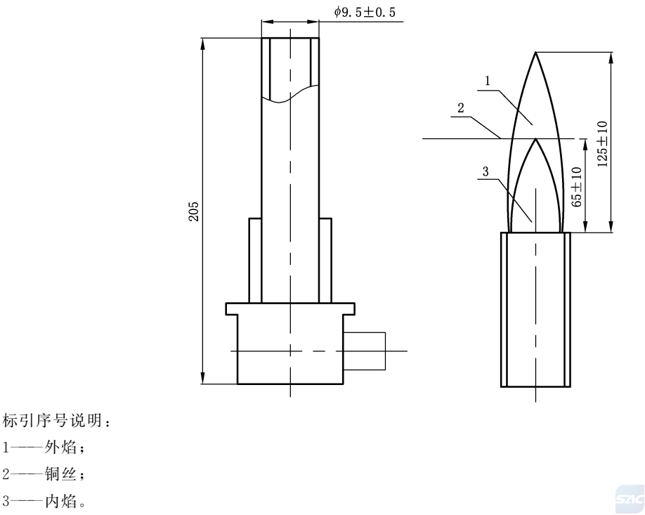
图 G.3 喷灯结构和喷灯火焰
