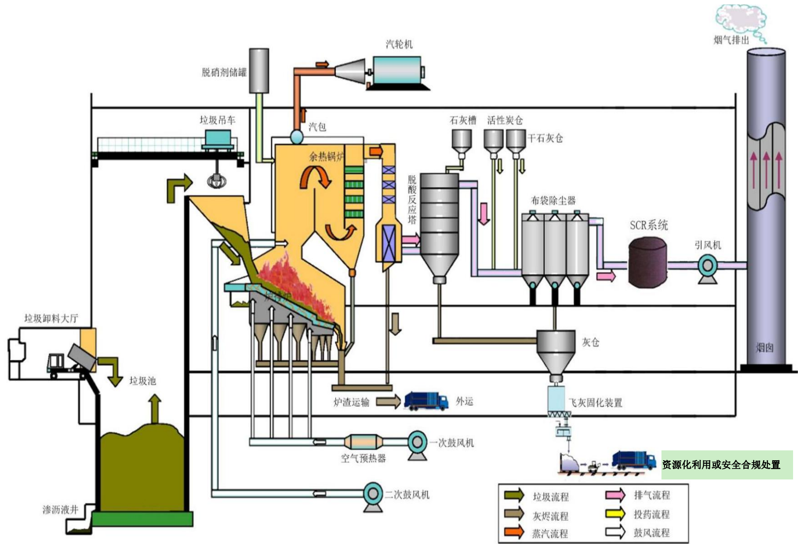
图 1 典型生活垃圾焚烧工艺流程
