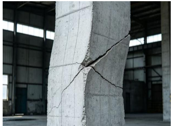
图 9.1.2-6 柱因刚度不足引起的挠曲侧弯变形
